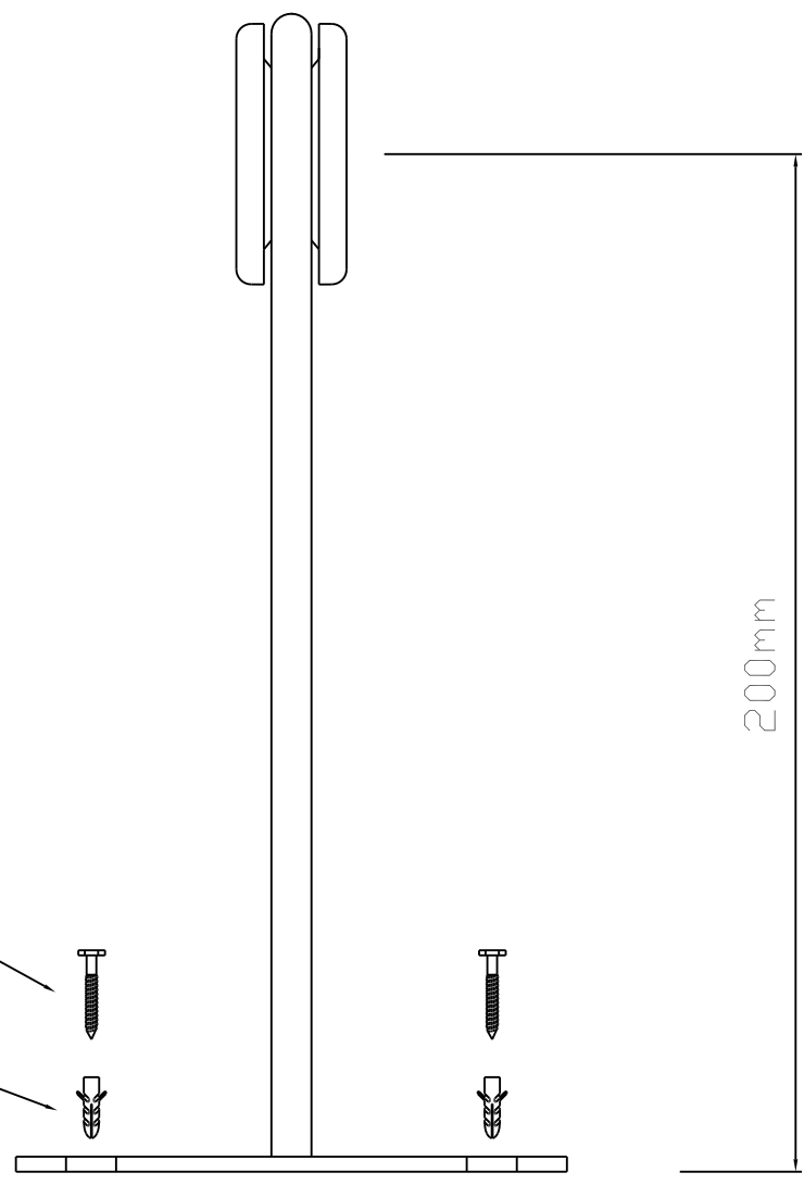
DETALHE DO ISOLADOR SIMPLES FIXAÇÃO HORIZONTAL - PRT201
