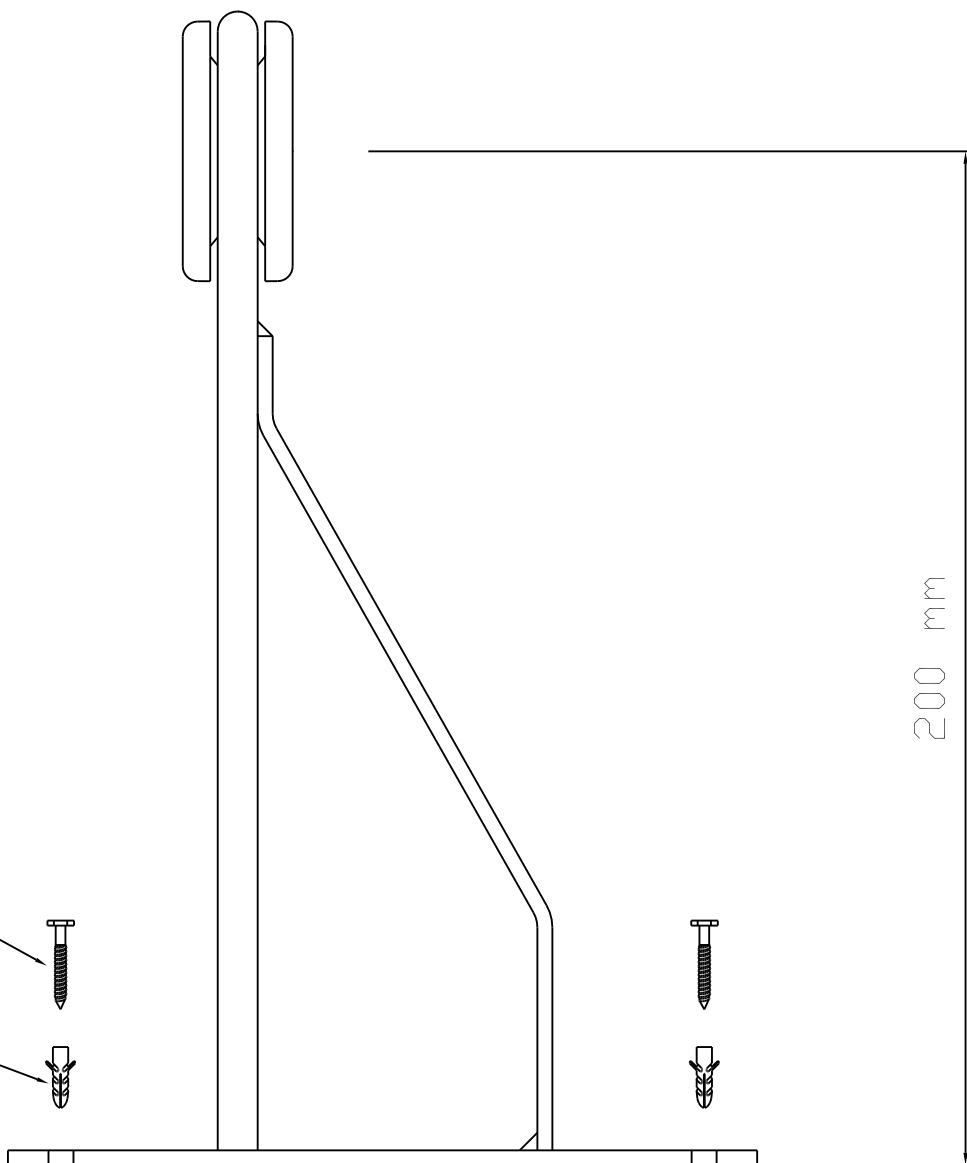
DETALHE DO ISOLADOR REFORÇADO FIXAÇÃO HORIZONTAL - PRT203
